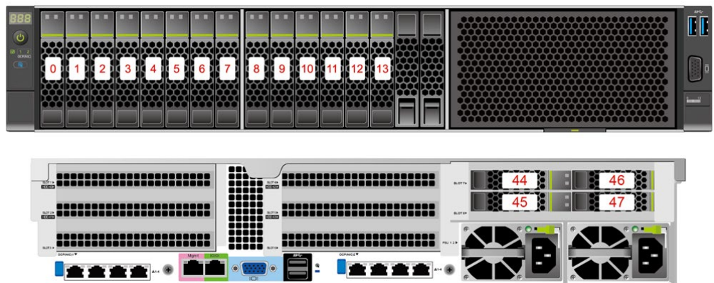
图3-19 8x2.5 SAS/SATA+6x2.5 NVMe 硬盘配置硬盘编号
