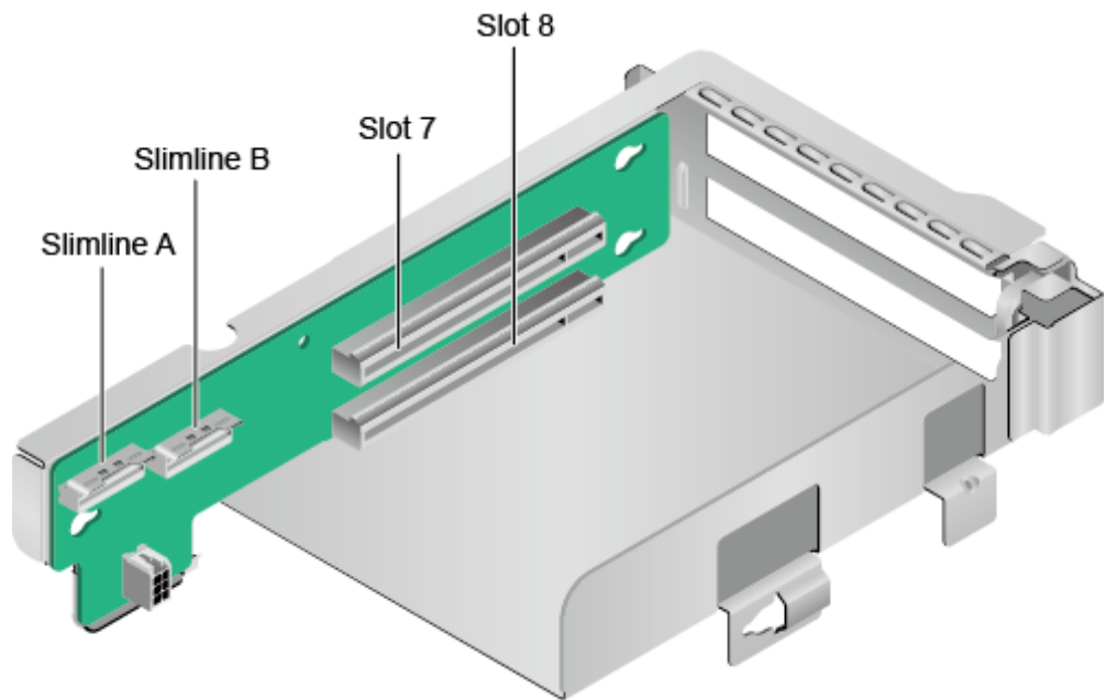
图3-31 Riser 卡 7 (2x8)
