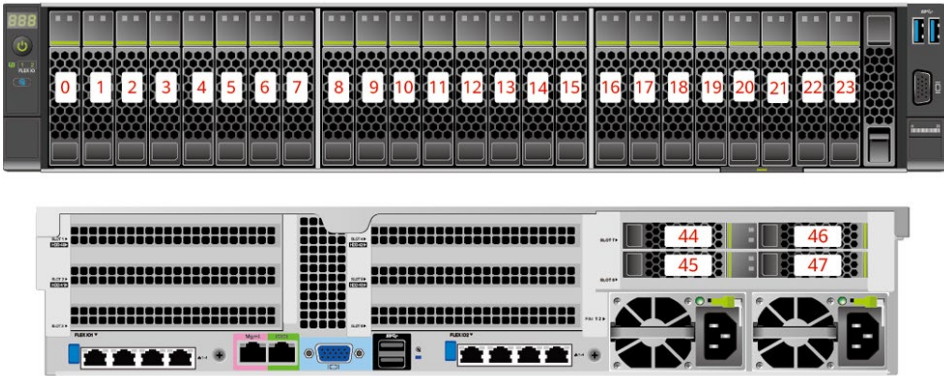
图3-16 24x2.5 英寸硬盘直通配置
