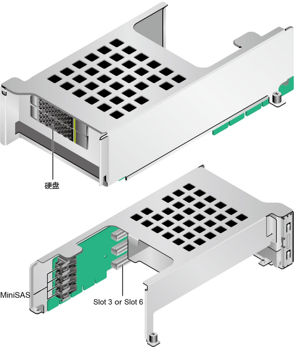
图3-30 Riser 卡 6（SAS Riser）（1）
