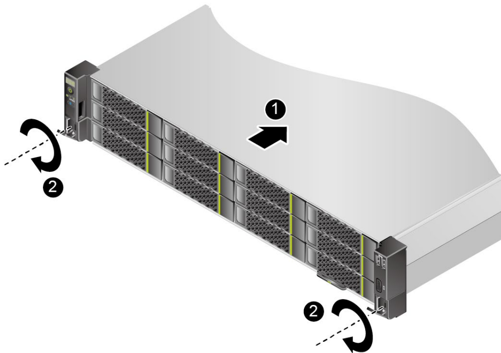
图6-9 安装服务器
