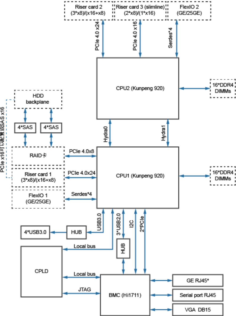
图2-3 逻辑结构
