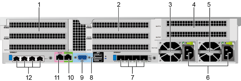
图3-8 后面板组件
