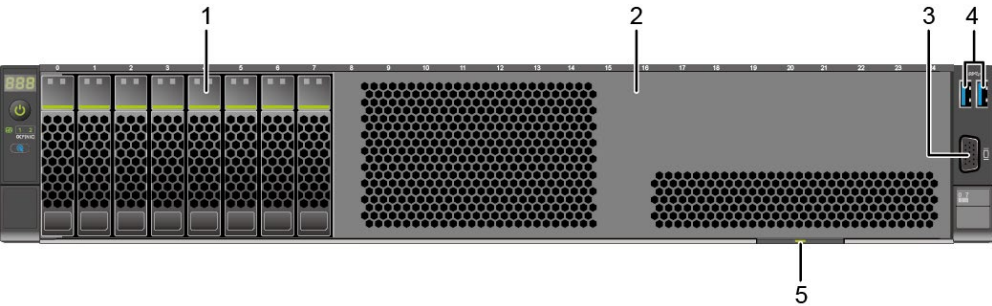
图3-6 8x2.5 英寸硬盘配置前面板组件
