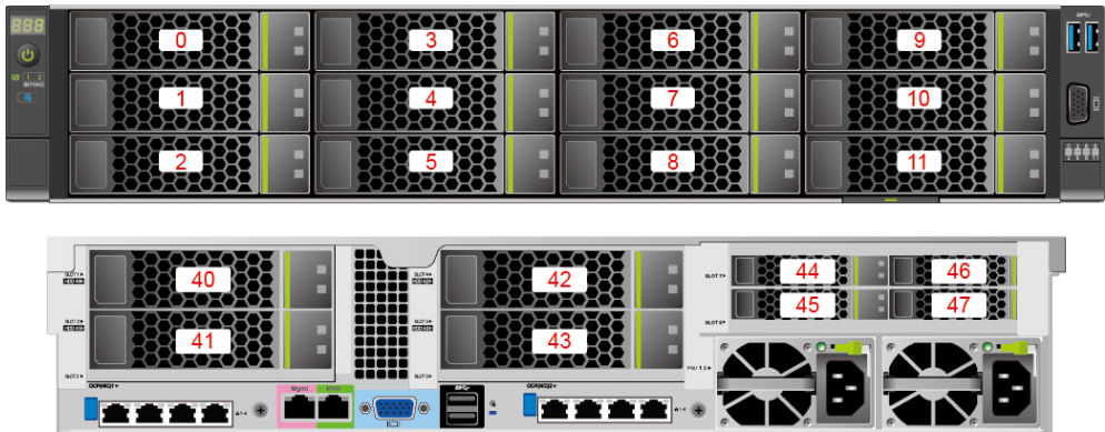
图3-12 12x3.5 英寸硬盘 EXP 配置硬盘编号
