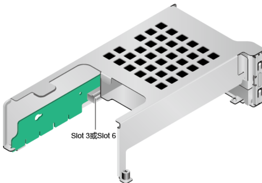
图3-29 Riser 卡 5 (1x16)
