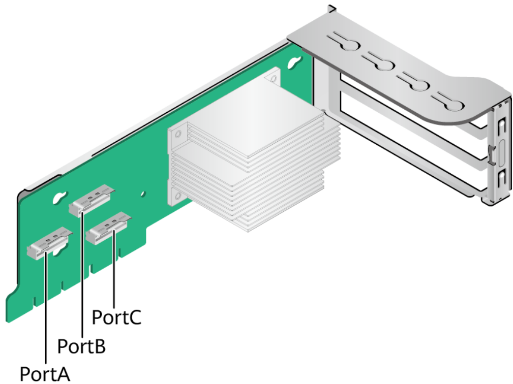
图3-27 Riser 卡 4
