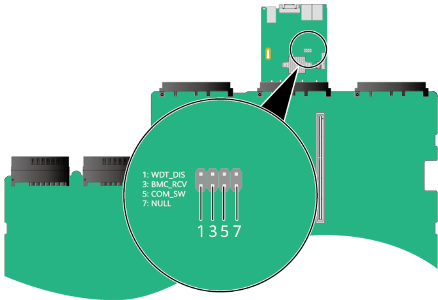
图8-13 跳线位置
