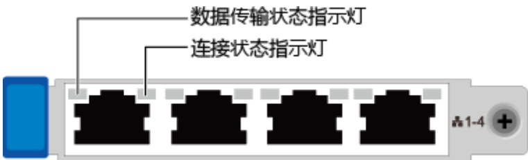
图3-10 TM210（4xGE 电口）
