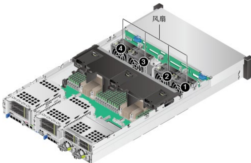
图3-34 风扇位置图
