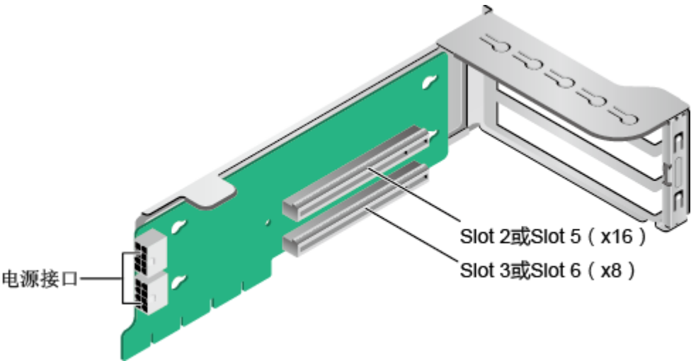
图3-25 Riser 卡 2（1x8+1x16）
