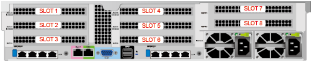
图3-33 PCIe 插槽
