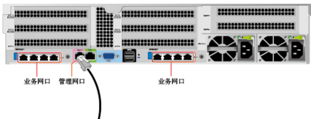
图6-11 连接网线
