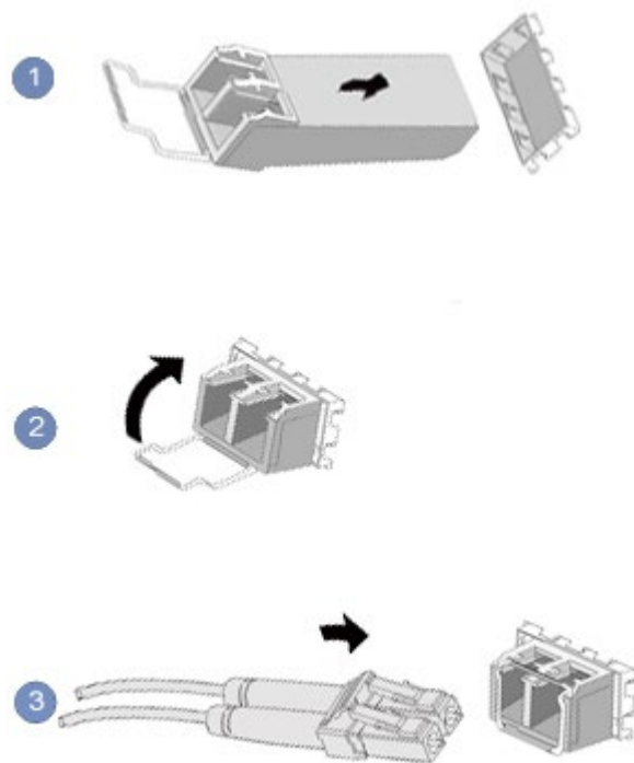
图6-12 连接光纤
