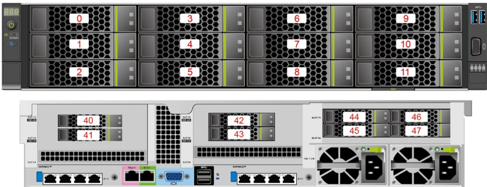
图3-14 12x3.5 英寸硬盘 RAID 直通配置
