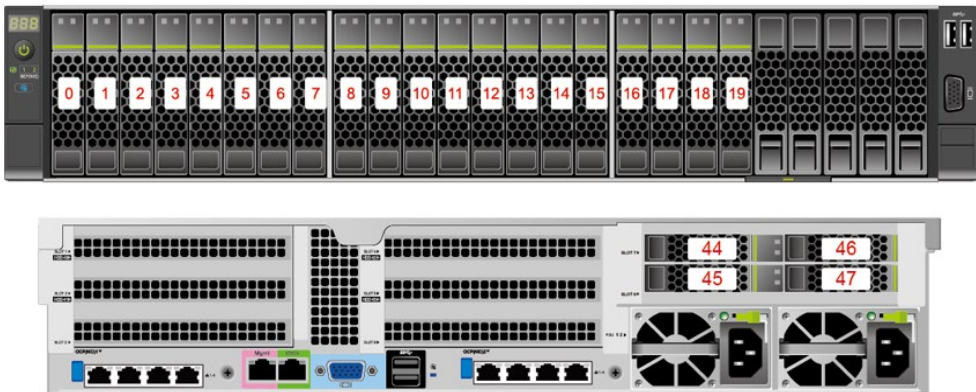
图3-18 8x2.5 SAS/SATA+12x2.5 NVMe 硬盘配置硬盘编号
