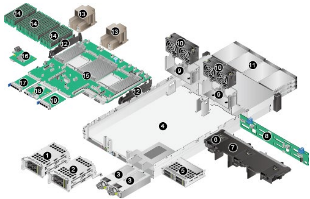
图2-2 部件
