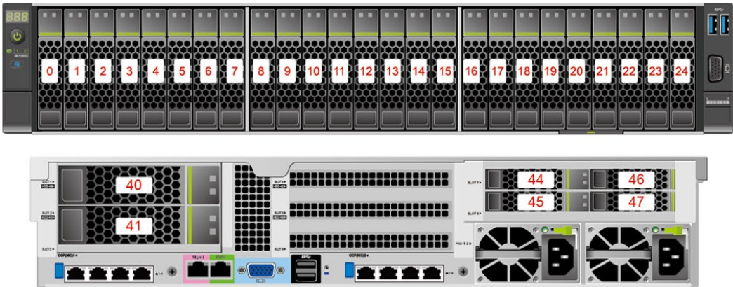
图3-15 25x2.5 英寸硬盘 EXP 配置硬盘编号
