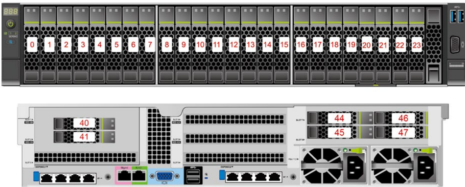
图3-17 24x2.5 英寸硬盘 RAID 直通配置的硬盘编号
