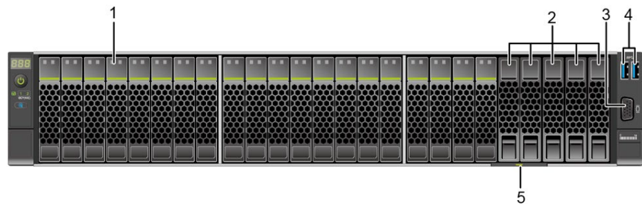
图3-4 8x2.5 SAS/SATA+12x2.5 NVMe 硬盘配置前面板组件
