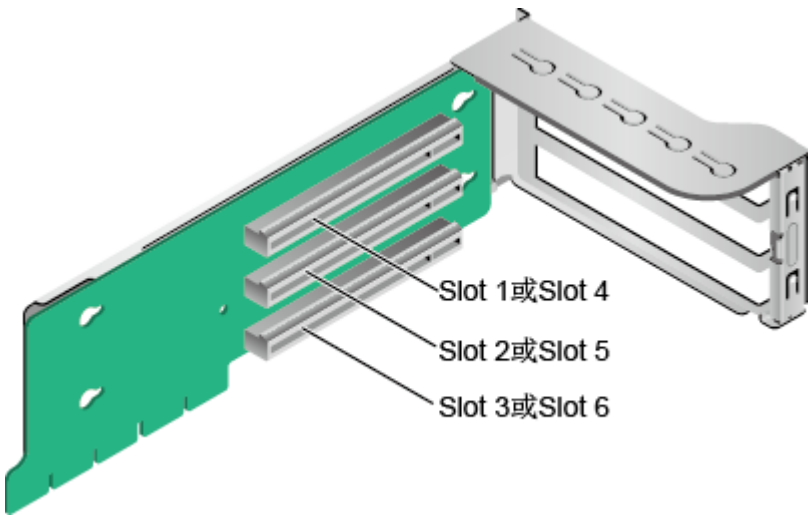
图3-24 Riser 卡 1（3x8）
