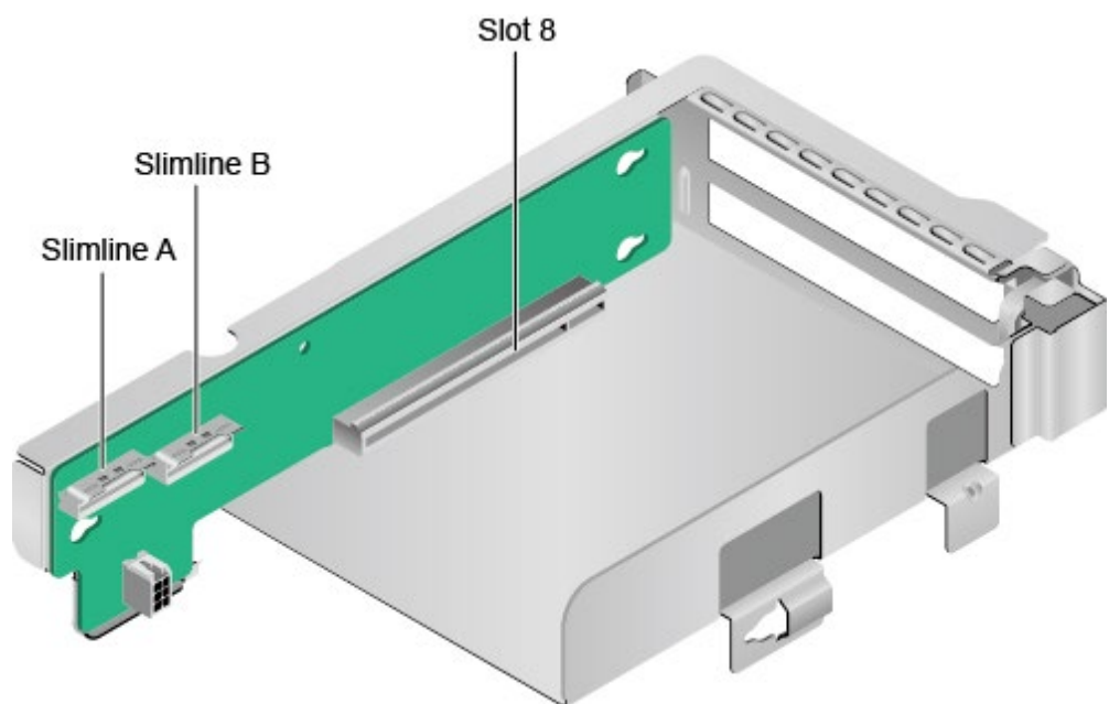
图3-32 Riser 卡 8 (1x16)
