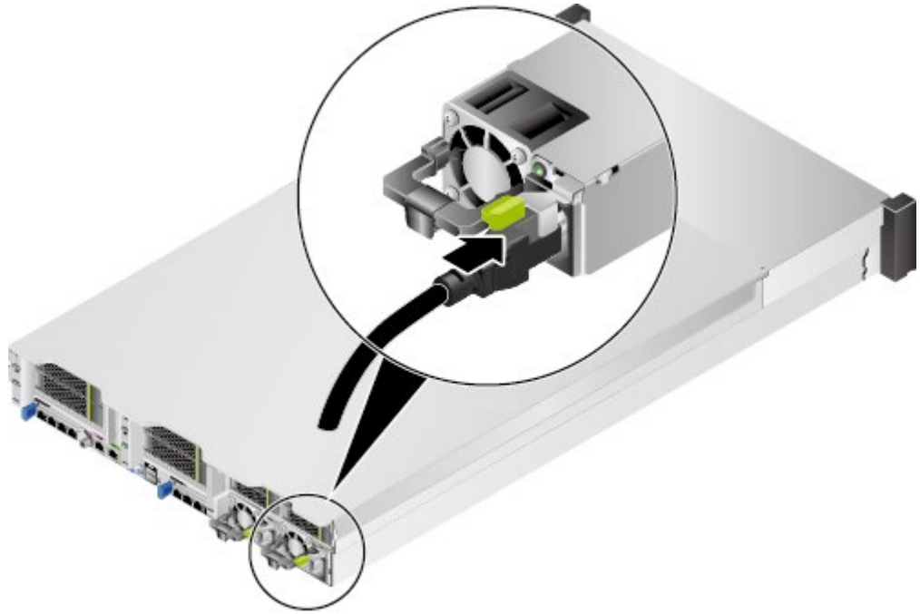
图6-17 连接电源线缆
