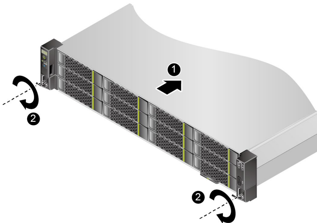
图6-7 安装服务器
