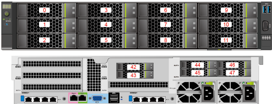
图3-13 12x3.5 英寸硬盘直通配置
