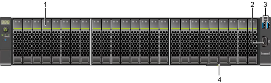
图3-2 25x2.5 英寸硬盘配置前面板组件
