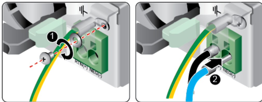
图6-19 连接线缆
