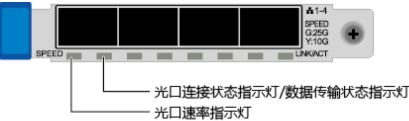
图3-11 TM280（4x25GE 光口）
