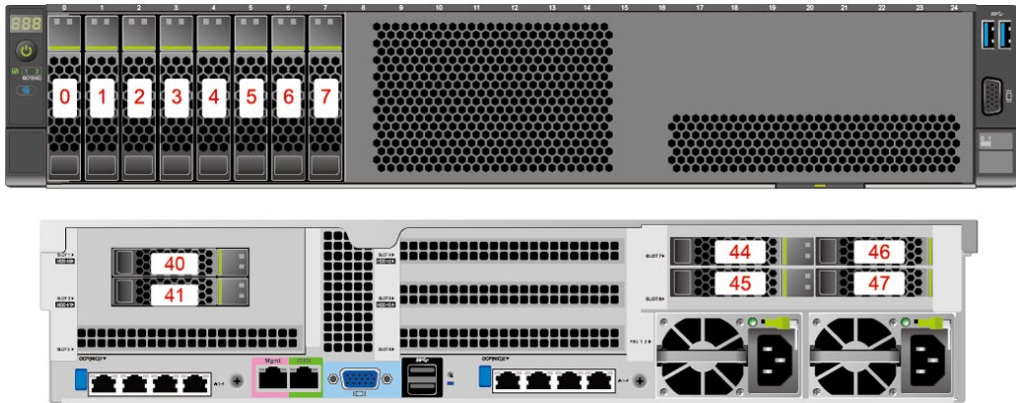
图3-21 8x2.5 英寸硬盘直通配置的硬盘编号
