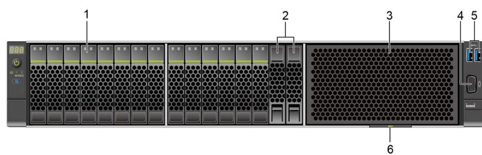
图3-5 8x2.5 SAS/SATA+6x2.5 NVMe 硬盘配置前面板组件
